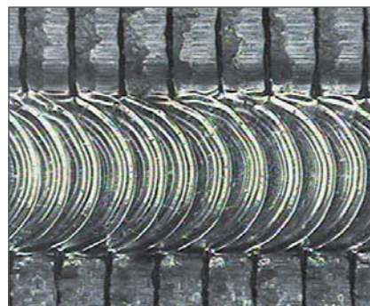
モーターコアシーム溶接 Motor core seam welding
