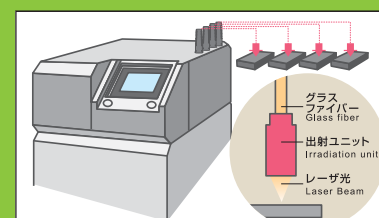
■ 6分岐対応図 Sharing of Maximum 6 (Option)
